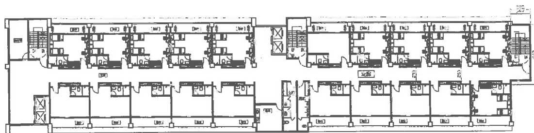
B棟 肆樓層平面圖 雙人宿舍-20間
