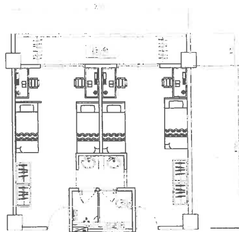
3 四人房平面配置圖 共計200間
