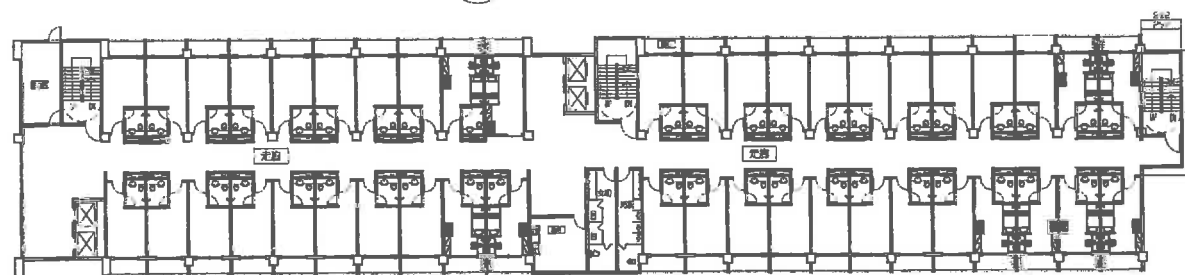
B棟 參樓層平面圖 雙人宿舍-5間 四大宿舍-15間
