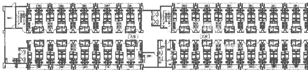
B棟 貳樓層平面圖 四人宿舍-22間
